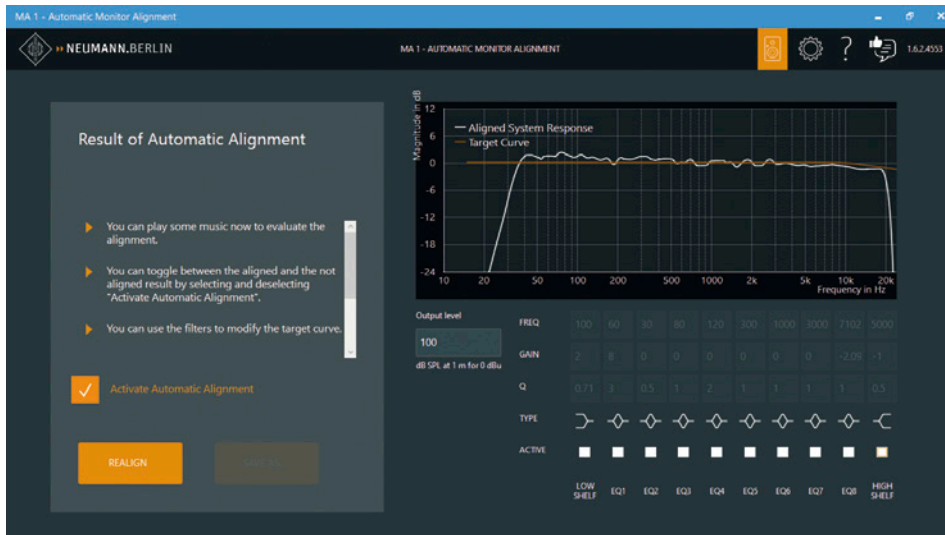
Abbildung 5 – Messergebnis inklusive Korrektur an der Hörposition für den Test
