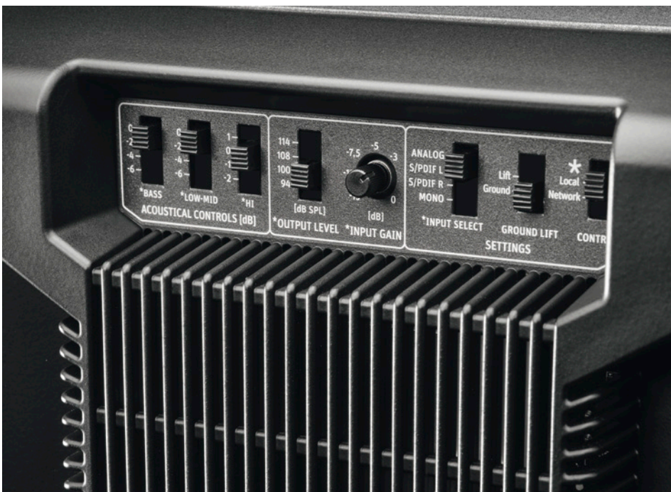
Der KH 150 verfügt über ein eigenes Bedienset für EQ, Ein- und Ausgangspegel, Eingangswahl, Groundlift und Netzwerk- oder Lokalbetrieb
