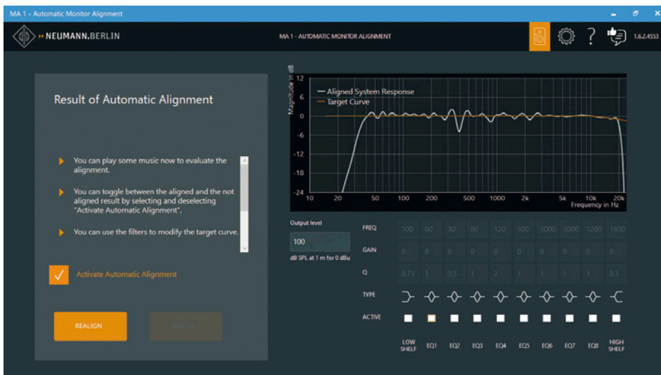
Abbildung 4 – Ergebnis einer Testmessung, die mit einem Multiband-EQ angepasst werden kann
